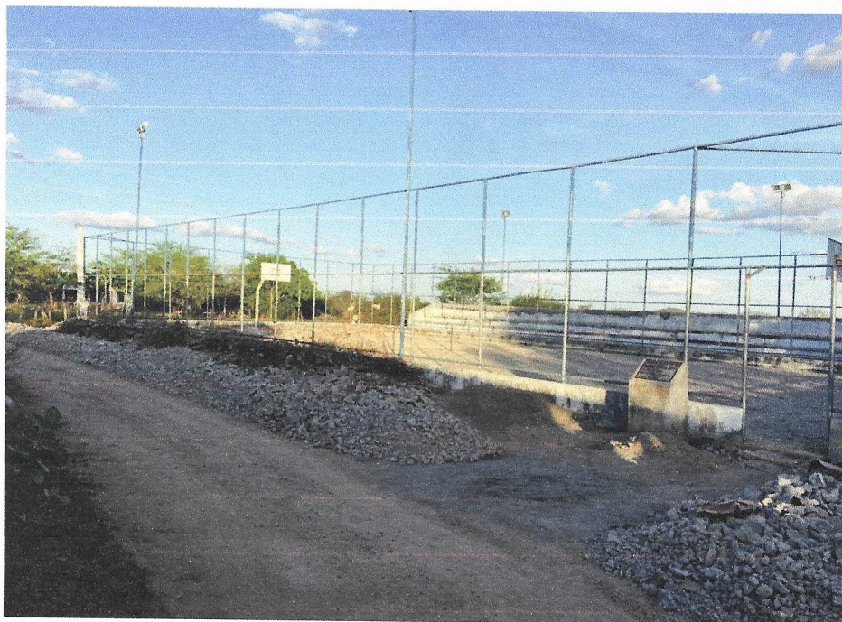
Foto 04 – Demolição de concreto com martelete e compressor
